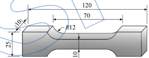
图 2 标准试件示意图(单位:mm)
